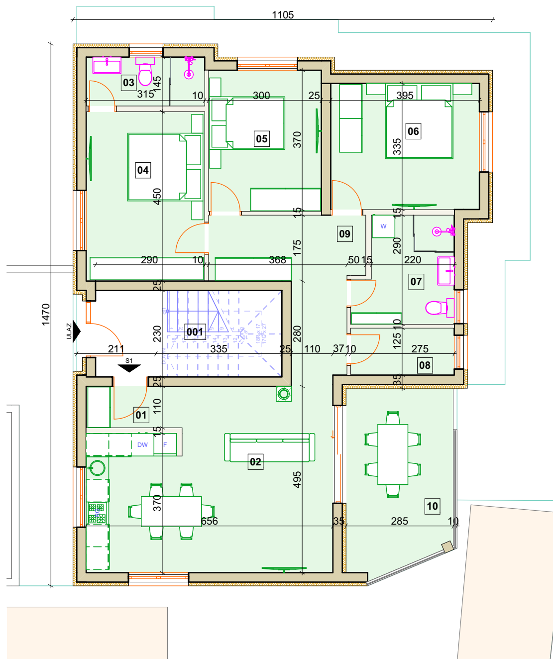
TLOCRT PRIZEMLJA
